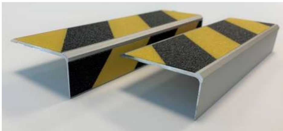
Beispiel: Treppenkanten 30 x 60 mm mit Einlage 50 mm gelb-schwarz beklebt, ohne und mit Setzstufenbeklebung mit 23 mm Einlage
